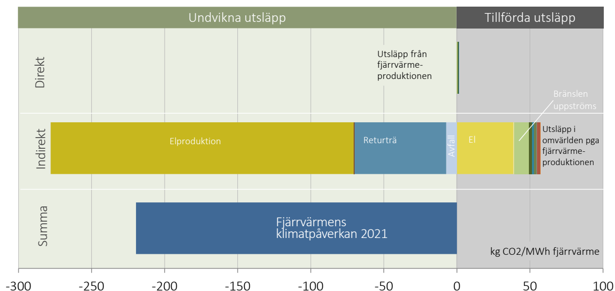
Figur 5 En fjärrvärmekunds klimatpåverkan under 2021 i Mölndal Energis fjärrvärmesystem. Den nedre blå stapeln "Fjärrvärmens klimatpåverkan 2021" är summan av tillförda utsläpp och undvikna utsläpp. Resultatet visar klimatpåverkan från att producera och leverera fjärrvärme fram till kund .
