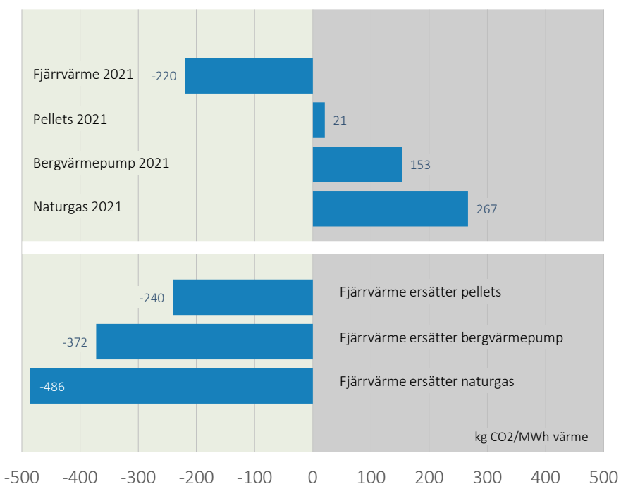
Figur 6 Klimatpåverkan för olika uppvärmningsalternativ 2021. I den övre delen av diagrammet jämförs en fjärrvärmekunds klimatpåverkan i Mölndal Energis fjärrvärmesystem med tre andra tekniker. I den nedre delen av diagrammet visas den resulterande klimatpåverkan då fjärrvärme ersatte någon av de andra uppvärmningsalternativen under 2021.
