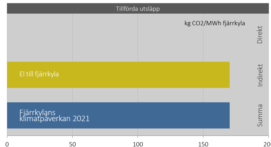
Figur 8 En fjärrkylakunds klimatpåverkan under 2021 i Mölndal. Den nedre blå stapeln "Fjärrkylans klimatpåverkan 2021" är summan av tillförda direkta och indirekta utsläpp. Resultatet visar klimatpåverkan från att producera och leverera fjärrkyla fram till kund .
