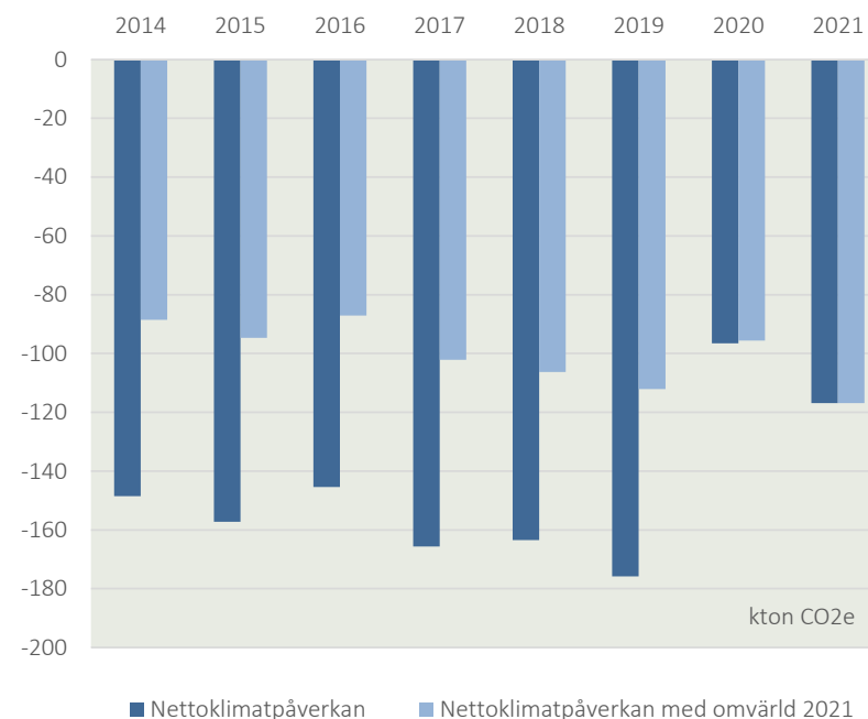
Figur 10 Klimatpåverkan för Mölndal Energi mellan åren 2014 och 2021. Figuren visar företagets klimatpåverkan för varje år med de omvärldsförutsättningar som då gällde samt för varje år med 2021 års omvärld. Detta belyser hur företagets utveckling påverkats av förändringar i företagets verksamhet och av förändringar i omvärlden
