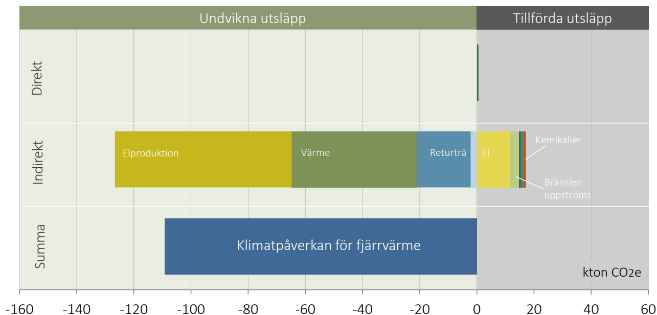
Figur 4 Fjärrvärmeproduktionens klimatpåverkan i Mölndal under 2021. Totalt bidrog fjärrvärmens till att undvika utsläpp motsvarande drygt 109 200 ton CO 2 e under 2021 (blå stapel).
