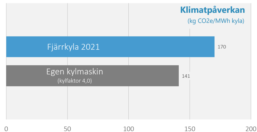
Figur 9 En fjärrkylakunds klimatpåverkan under 2021 i Mölndal i jämförelse med en ny egen kylmaskin.
