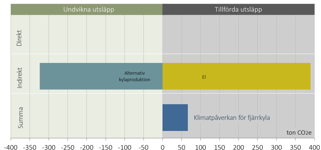
Figur 7 Fjärrkylaverksamhetens klimatpåverkan i Mölndal under 2021. Totalt bidrog fjärrkylan till ett utsläpp motsvarande 66 ton CO 2 e under 2021 (blå stapel).
